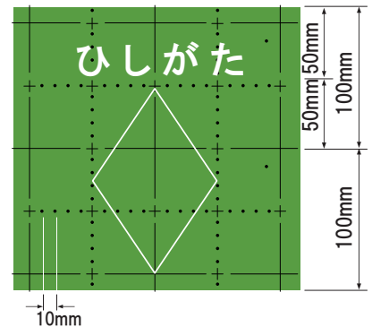
暗線プリント（焼成）パターンと使用例
